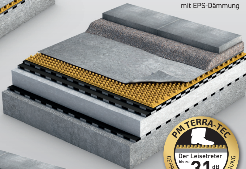
Warmdachaufbau mit EPS-Dämmung
